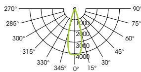
2x20° (1/10)
